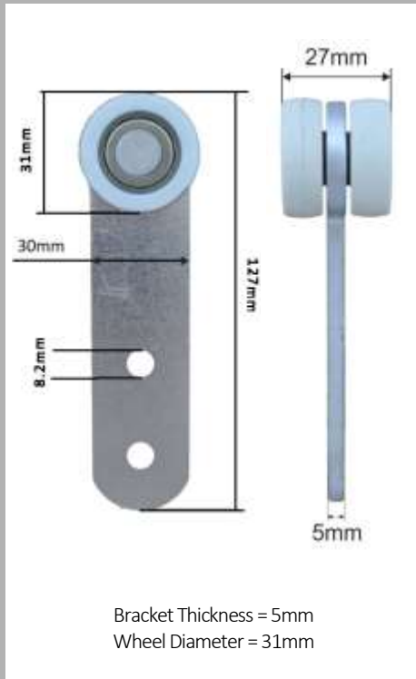
D31mm x W27mm = Part No: 113784
