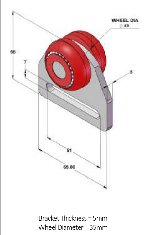
D35mm x W31mm = Part No: 113772 D35mm x W34mm = Part No: 113777
