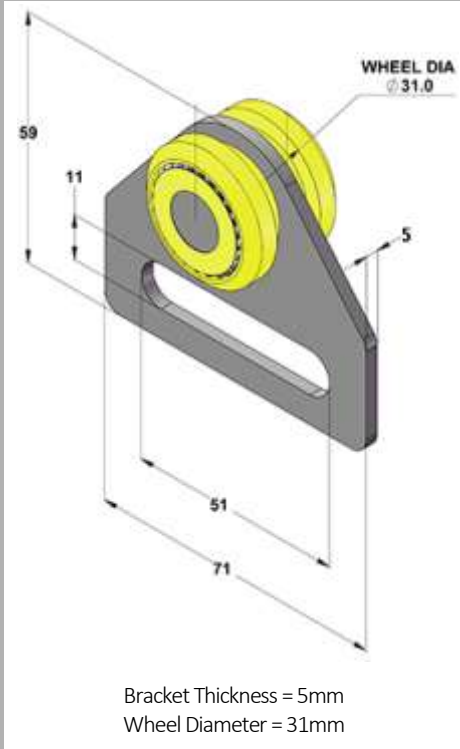
D31mm x W30mm = Part No: 113768 D31mm x W31mm = Part No: 113756
