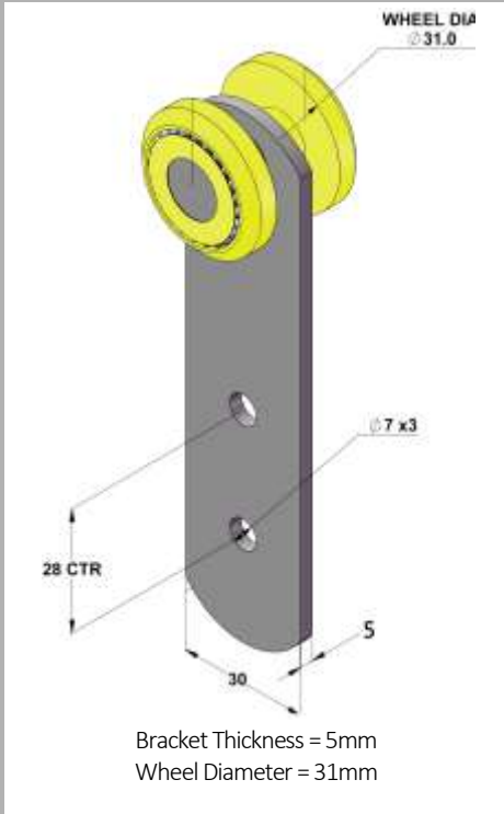
D31mm x W27mm = Part No: 113776 D31mm x W30mm = Part No: 113769 D31mm x W33mm = Part No: 113778 D31mm x W38mm = Part No: 113755
