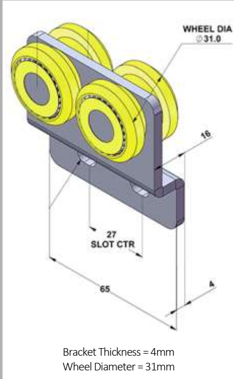
D31mm x W25mm = Part No: 113813
